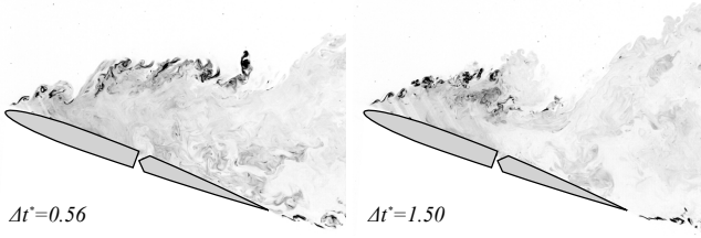
Figure 8: \alpha_{LE} = 20^\circ , \delta = 20^\circ \rightarrow 21^\circ , 6Hz
