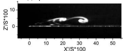
(d) A-A sectional view of the helical vortex
